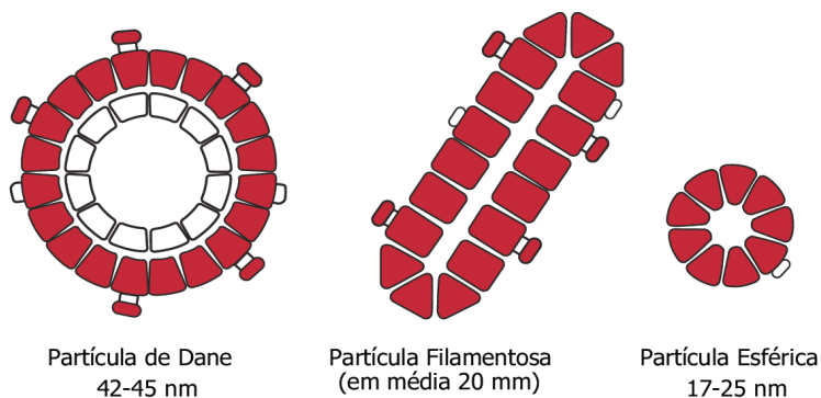
Figura 8. Representação esquemática da estrutura das partículas virais e subvirais do vírus da hepatite B (HBV)
