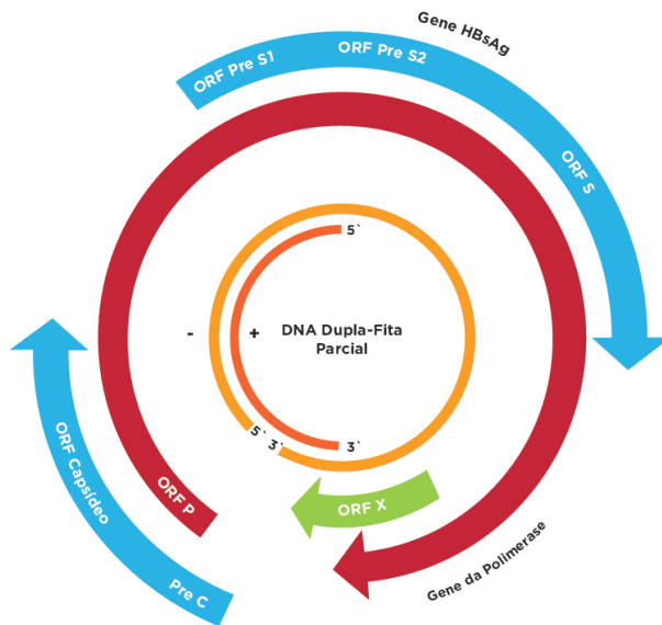
Figura 6. Representação esquemática da organização genômica do vírus da hepatite B (HBV)
