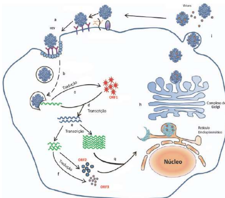
Figura 21. Ciclo replicativo do vírus da hepatite E (HEV)
